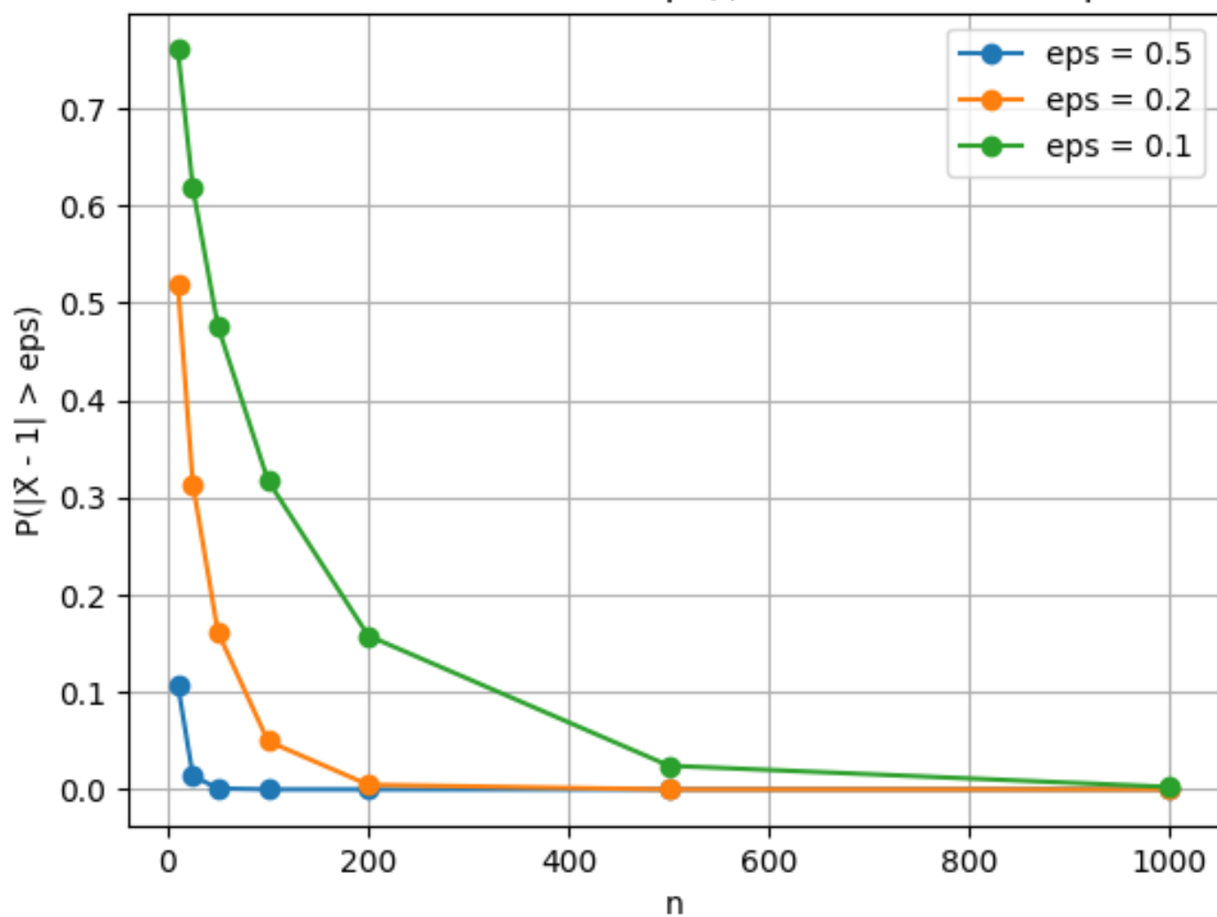
Состоятельность \bar{X} по определению (монте-карло)
