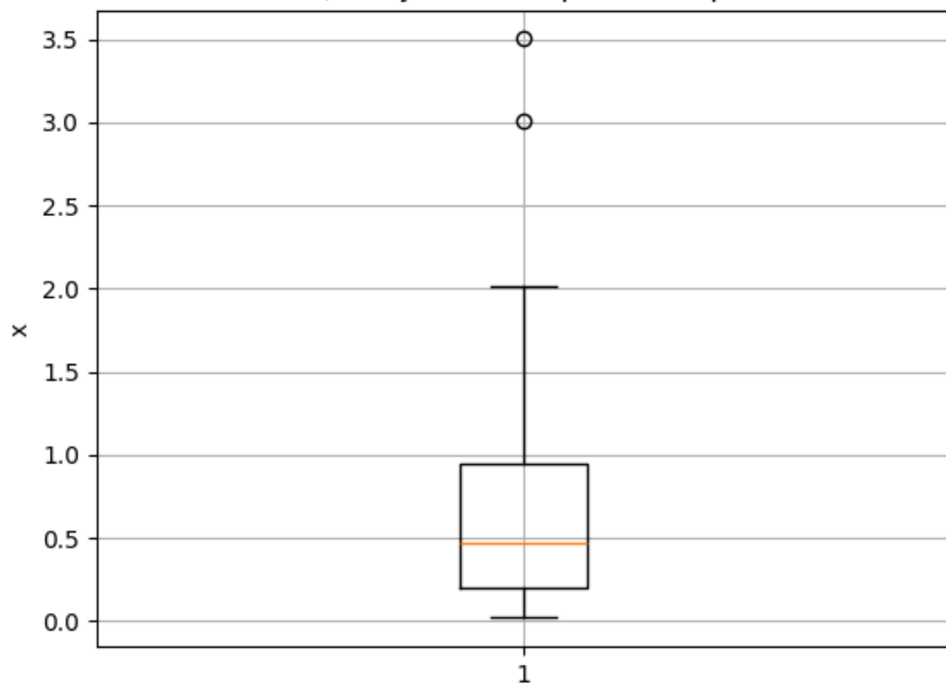
Ящик с усами (boxplot) выборки
