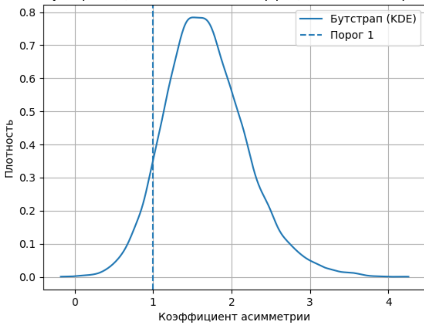
Бутстрап-оценка плотности коэффициента асимметрии
