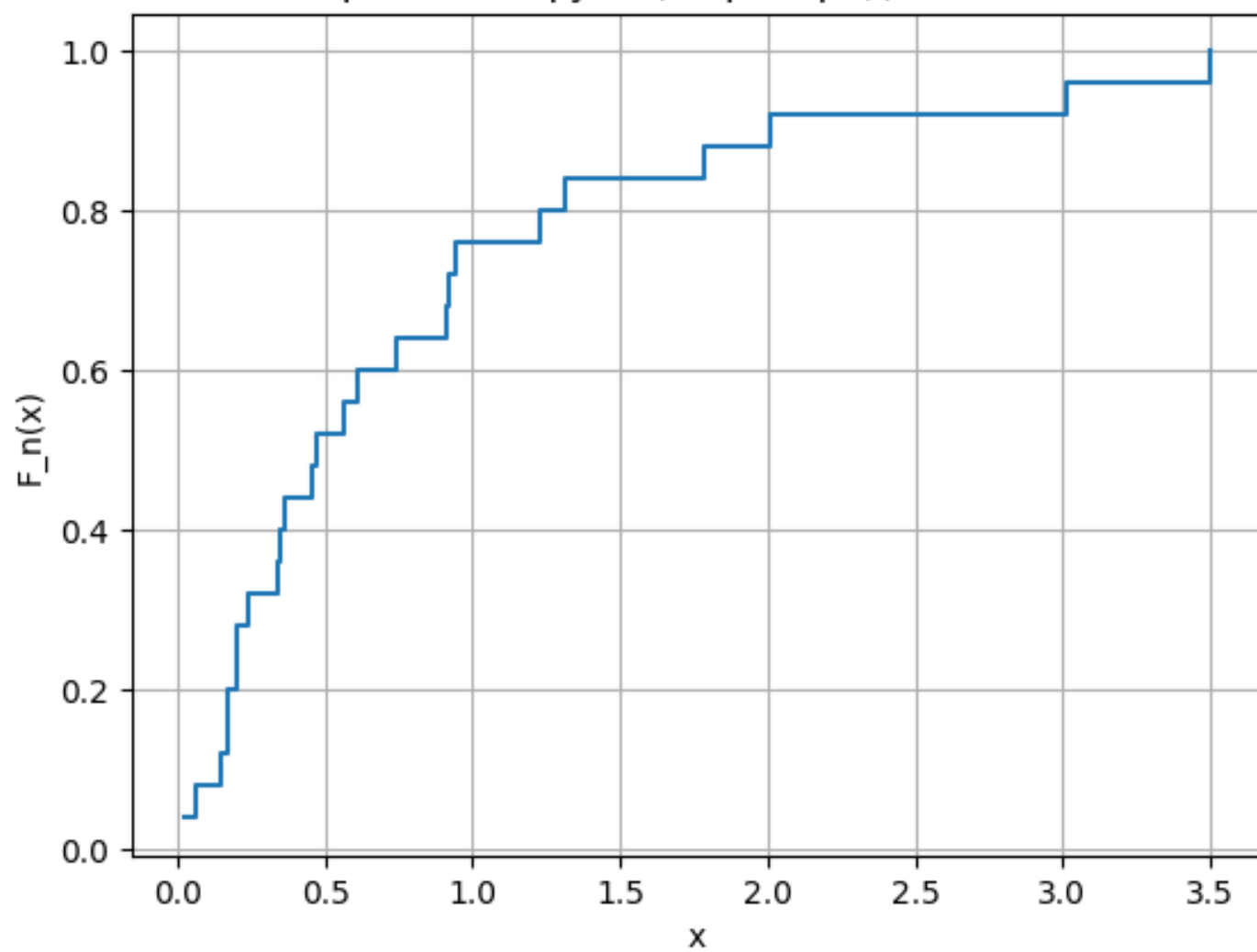
Эмпирическая функция распределения (ЭФР)
