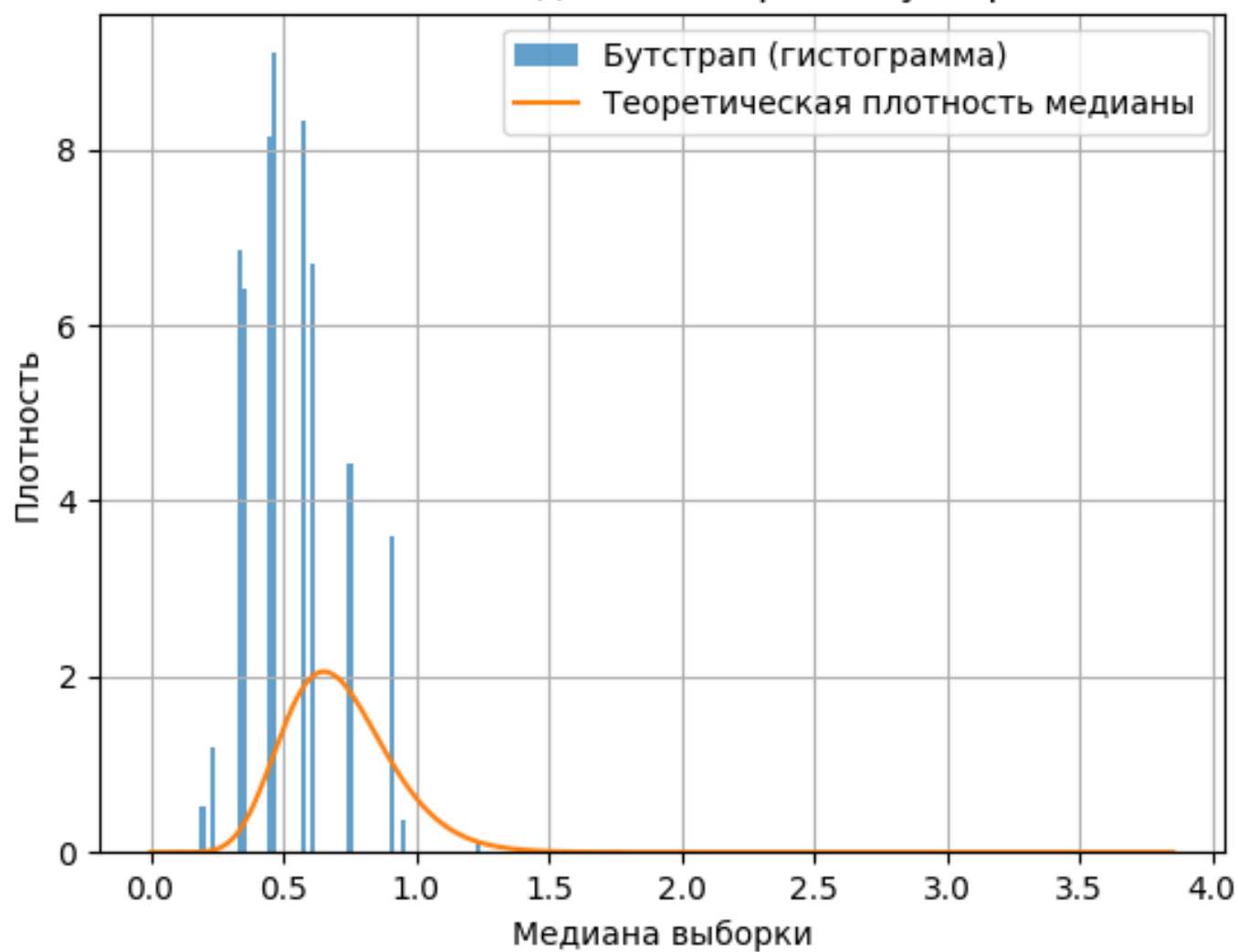
Плотность медианы: теория и бутстрап
