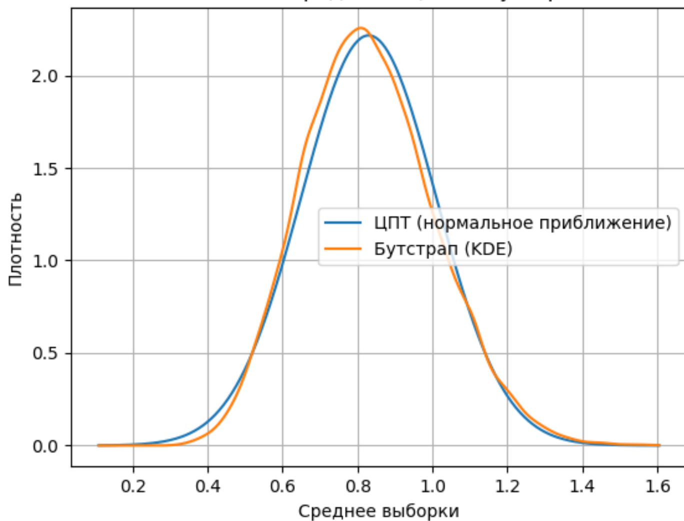
Плотность среднего: ЦПТ vs бутстрап
