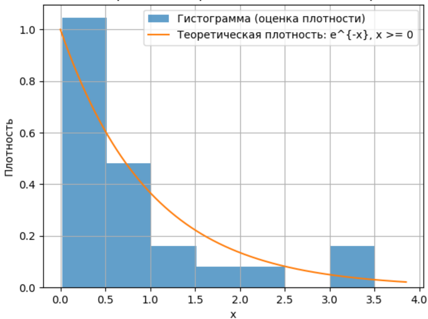
Гистограмма и теоретическая плотность Exp(1)
